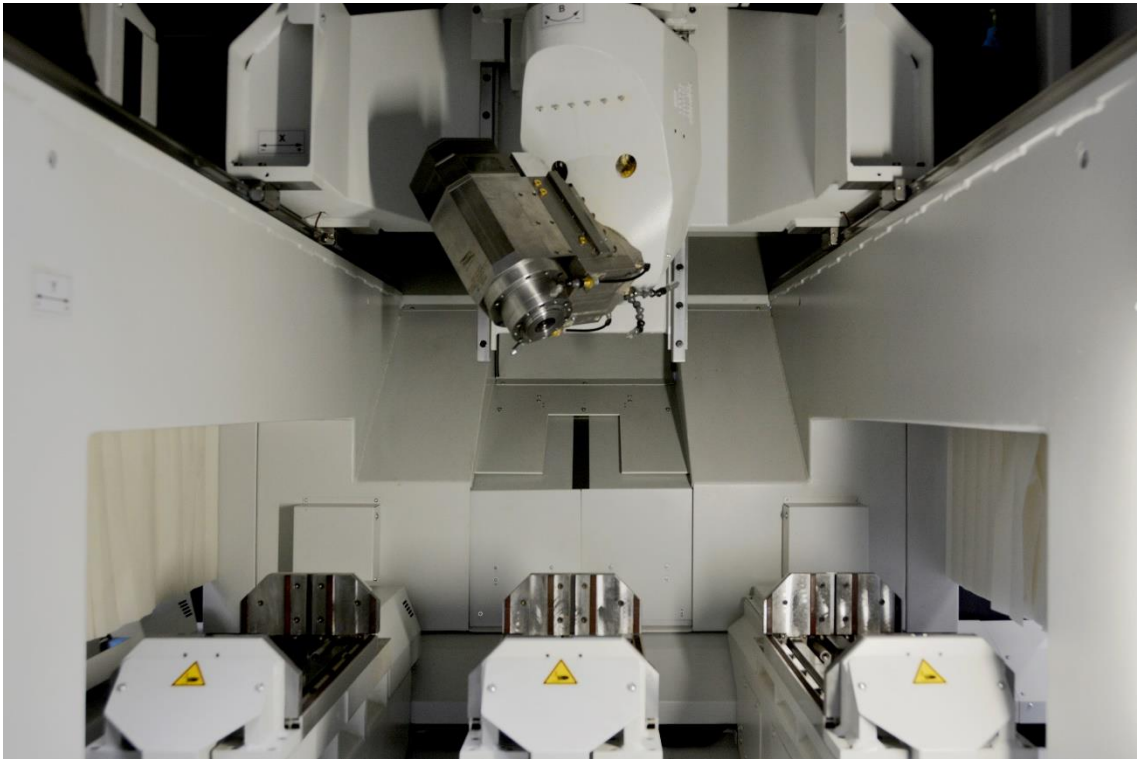
Kühlstrahl- und Schmiergerät, das zum Bearbeiten von Aluminium ein Öl-/Luftgemisch an die Schneide bläst.
