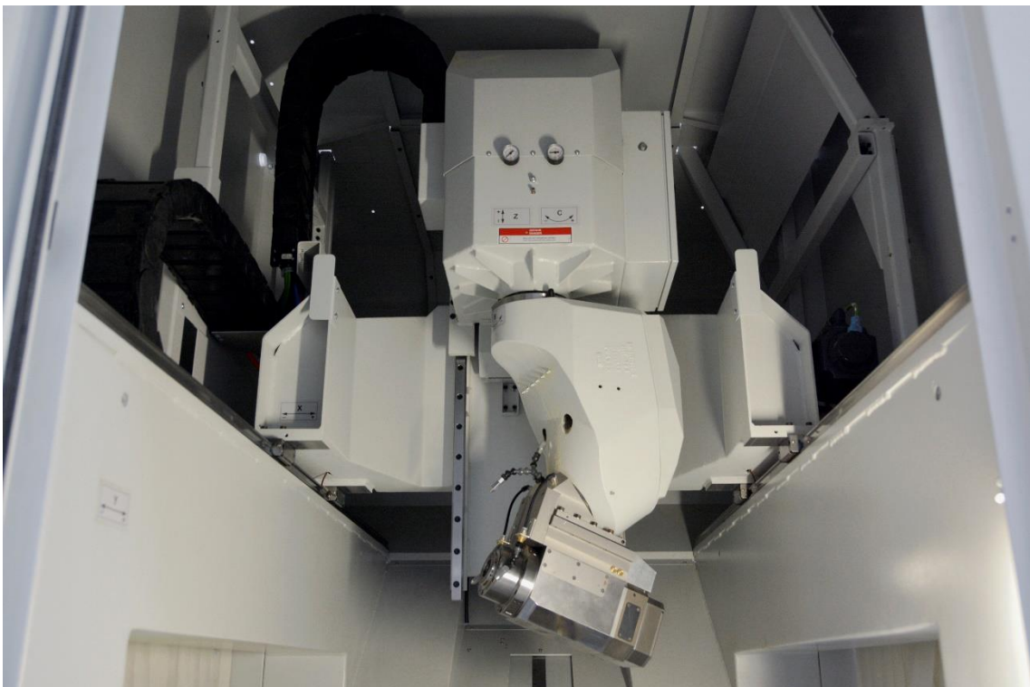
Kardanischer Arbeitskopf mit 35 kW Frässpindel für Fräs-, Bohr-, Säge- und Schleifarbeiten. 20° unterschwenkend.
