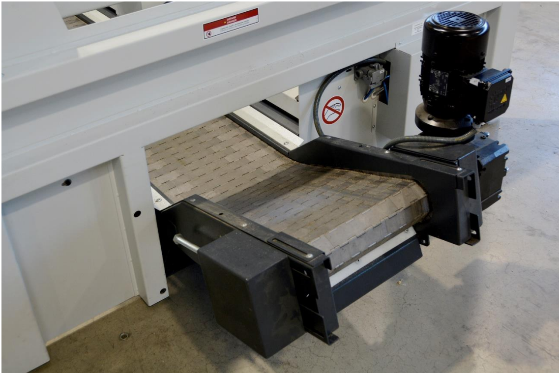
Scharnierbandförderer, der die Späne in X-Richtung nach rechts aus dem Maschinenbett transportiert.
